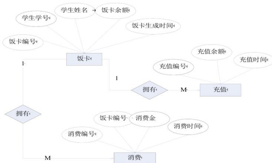
图 2.3.1 E-R 图
