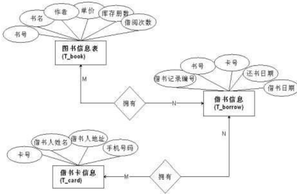
图 2.15.1 E-R 图
